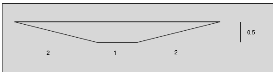
Figur 36: Principskiss över dikessektion längs med den södra planområdesgränsen
