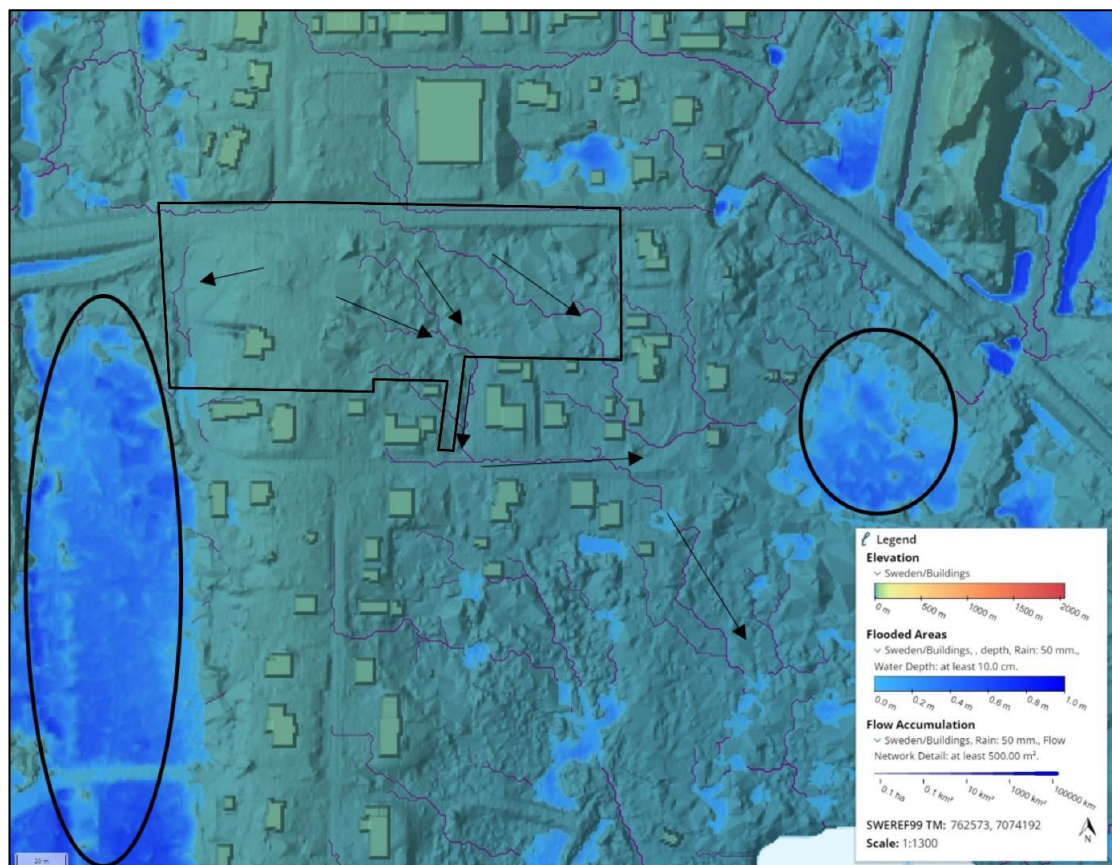
Figur 30. Befintliga avrinningsstråk inom och i anslutning till planområdet. Planområdet är markerat med svart och svarta pilar indikerar de huvudsakliga avrinningsvägarna. Inringade områden markerar lågpunkter dit vatten från planområdet avleds vid skyfall (WSP, 2023).
