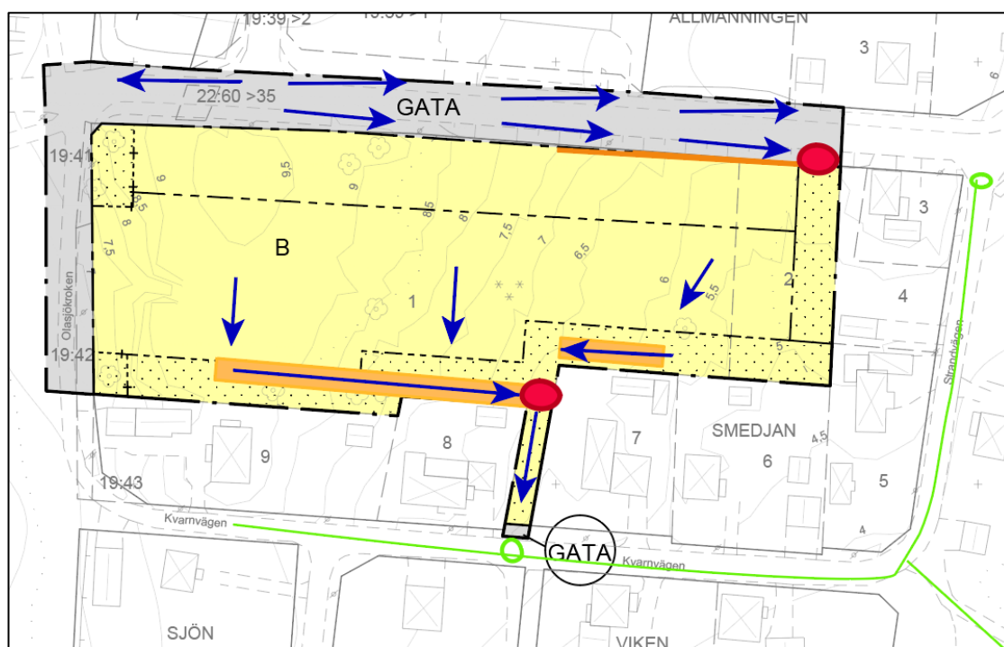
Figur 35: Översikt över föreslagen dagvattenlösning inom planområdet. Orange symboliserar dagvattendiken. Röd cirkel symboliserar möjlig placering av kupolbrunn i dike och vidare avledning till det kommunala ledningsnätet. Föreslaget dike är markerad i orange längs med Linjevågen. Illustration redigerad av Umeå kommun efter färdig plankarta.
