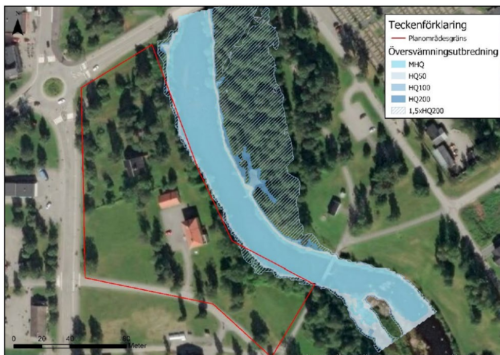
Figur 39. Illustration från översvämningstudien (2021). Översvämning utbredning vid högflöden med olika återkomsttid vid medelvattenstånd. Notera att för flödet som är 1,5 gånger större än HQ200 finns ingen beräknad återkomsttid.
