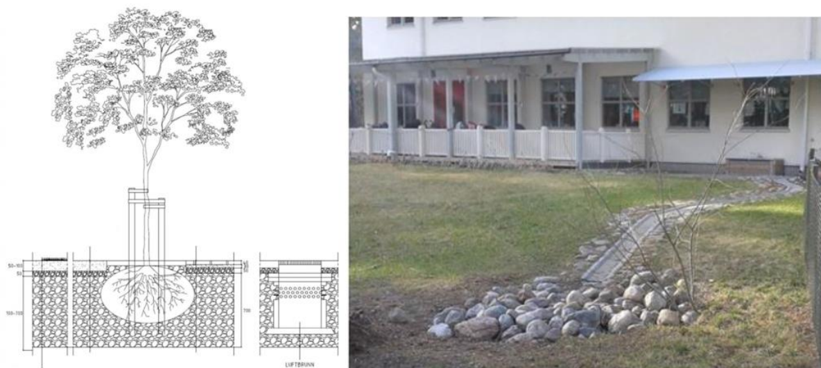
Figur 26. Till vänster: En principskiss på uppbyggnad av skelettjord under träd. Bilden är hämtad från Bara Mineralers hemsida. Till höger: Exempel på en hårdgjord rämma som leder takvattnet till en liten stenkista. Bilden är tagen i Gävle.
