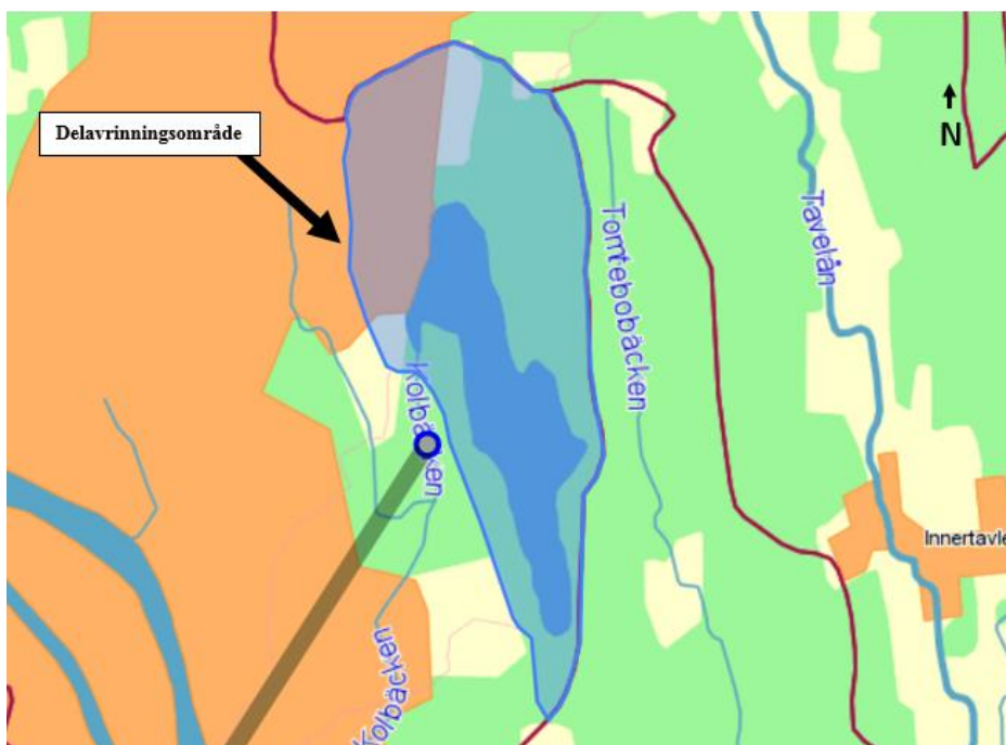
Figur 8. Delavrinningsområde till Nydalasjön som innefattar planområdet redovisat i transparent blå färg. Bildkälla: SMHI 2018.
