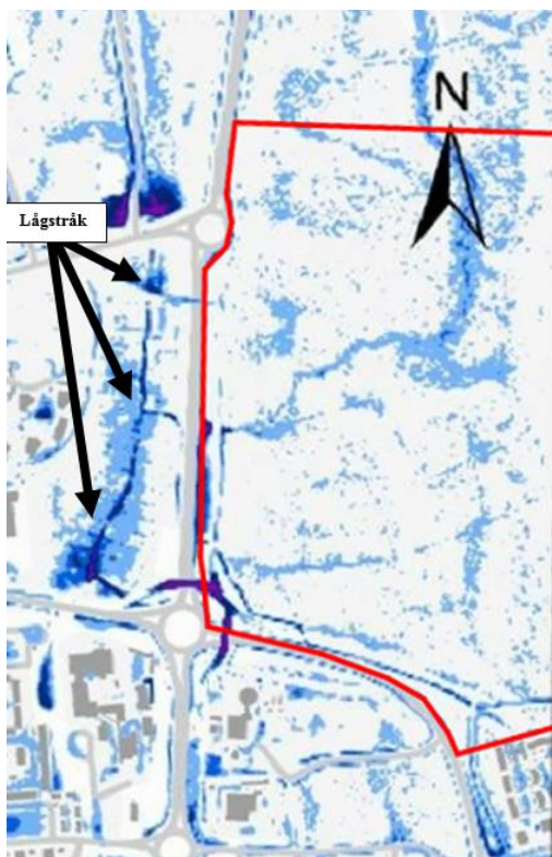
Figur 10. Skyfallsanalys som visar översvämningssytor väster om planområdet. Planområdet är markerat i rött. Bildkälla: "Skyfallskartering Västerbottens län, Umeå kommun" Länsstyrelsen i Västerbottens län, april 2018.
