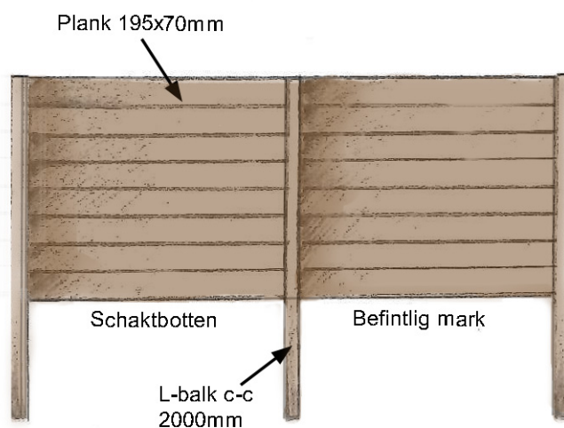
Figur 3. Skyddsspont.
